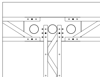
TT Configurazione angolo moduli TL30-TL22-TL30 .
